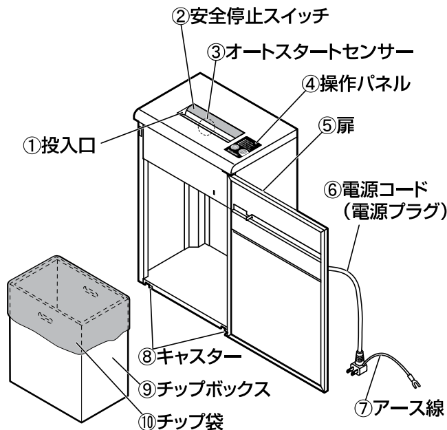
図1 外観図
