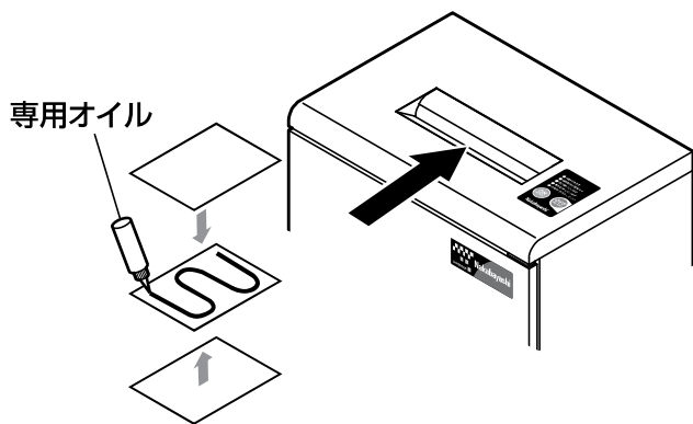
図6 注油方法
